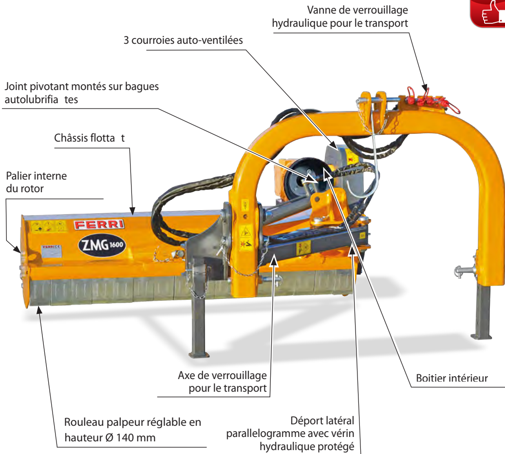
Le vérin de mouvement hydraulique se trouve à l'intérieur des bras du parallélogramme.
