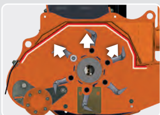
Tôle de blindage interne "Full Coverage" en Domex 700.
