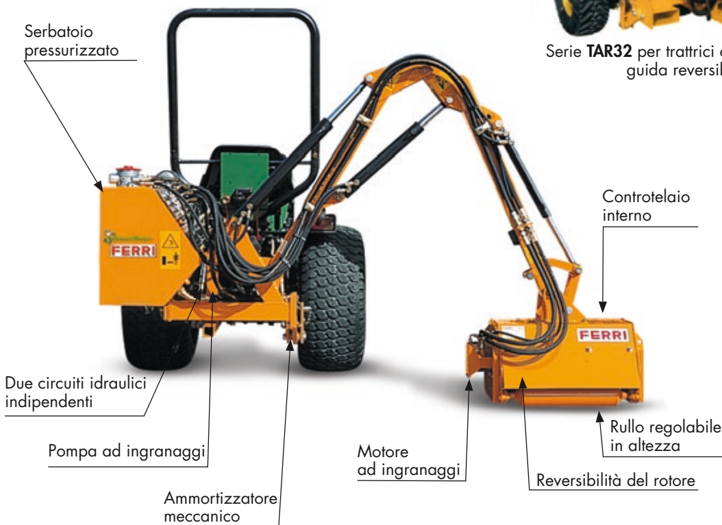
Sistema Floating
